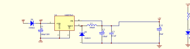
电源部分
